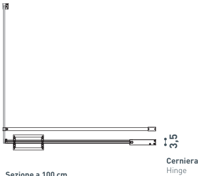
Sezione a 100 cm Section at 100cm
