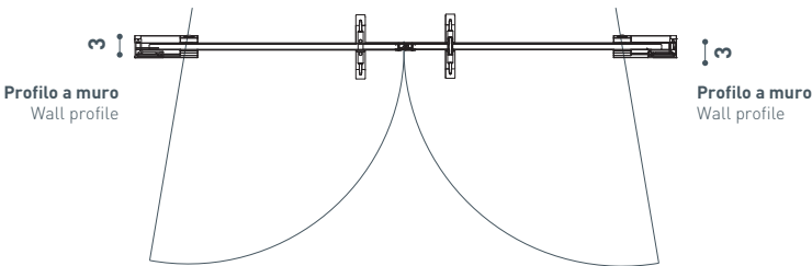
Sezione a 100 cm Section at 100cm
