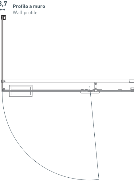
Vista dall'alto. Top view
